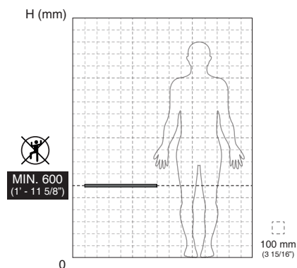
Sicherheitsabstand
