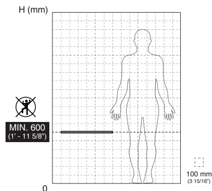
Расстояния безопасности
