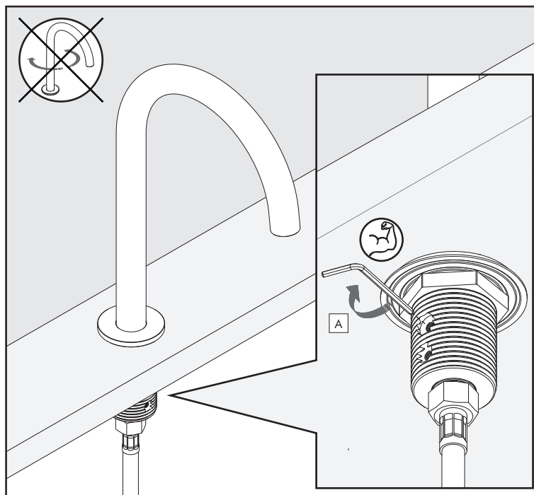
FISSAGGIO OPZIONALE BOCCA DI EROGAZIONE / SPOUT OPTIONAL FIXING / OPTIONALER BEFESTIGUNG DES AUSLAUF / FIJACIÓN OPCIONAL DE CAÑO / OPTION DE FIXATION DU BEC
