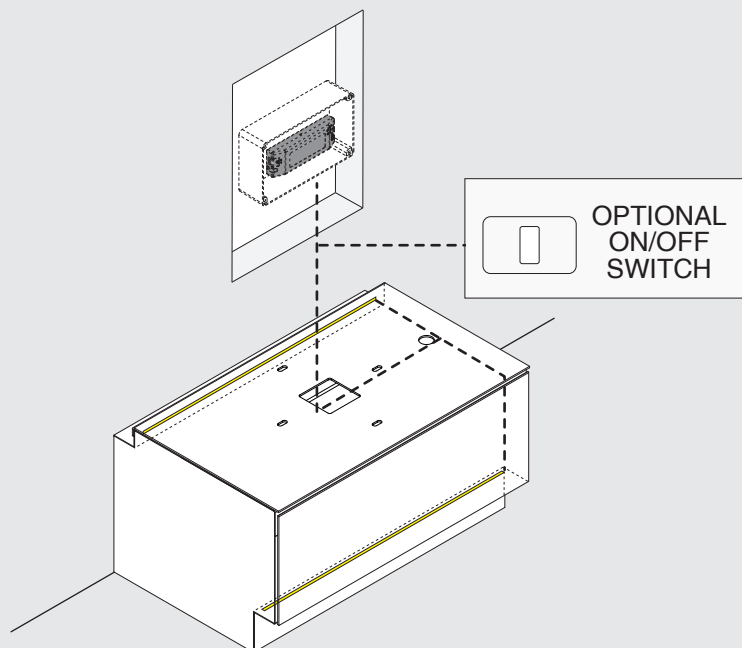
A Allumer/éteindre les lumières de courtoisie avec bouton à distance
