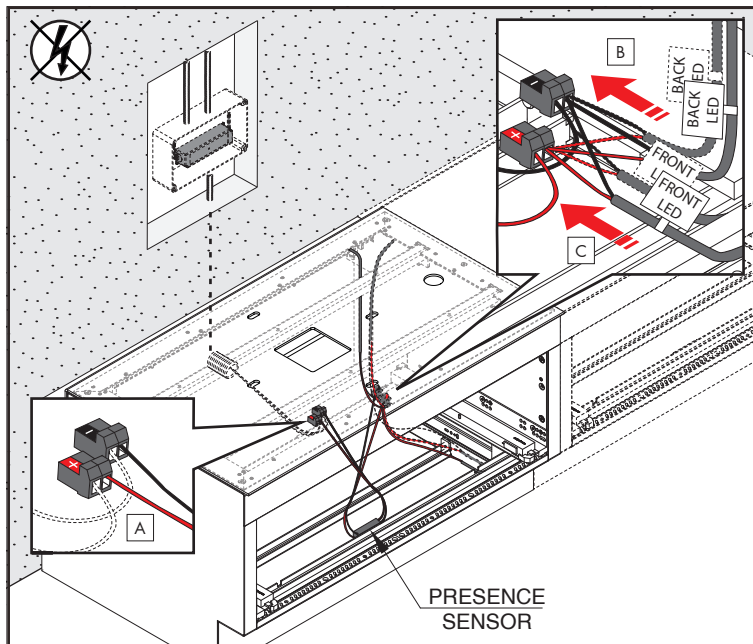
7B Accensione / spegnimento luci di cortesia con rilevatore di presenza On / off courtesy light with presence sensor
