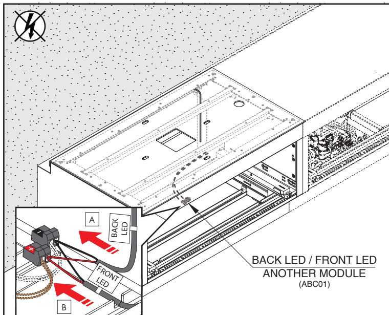
7B Accensione / spegnimento luci di cortesia con rilevatore di presenza On / off courtesy light with presence sensor
