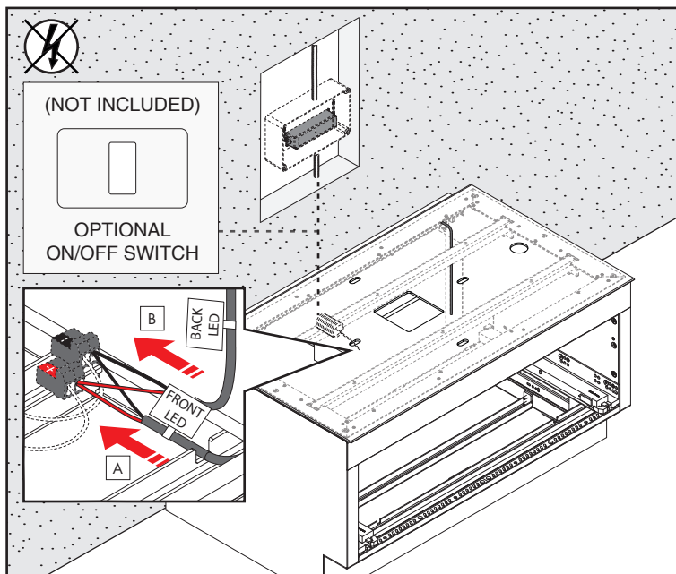
9A Accensione / spegnimento luci di cortesia tramite pulsante remoto On / off courtesy light with remote control
