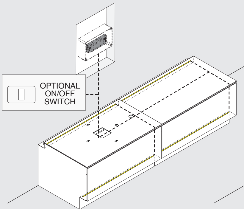
A Accensione / spegnimento luci di cortesia con pulsante remoto
