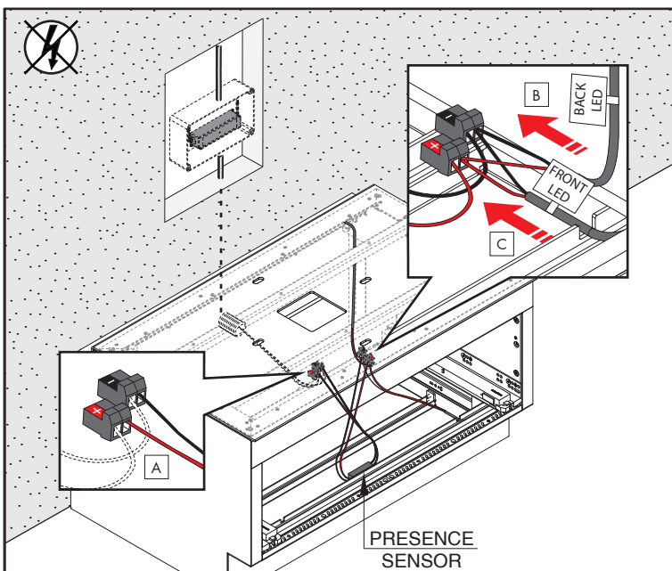
9B Accensione / spegnimento luci di cortesia con rilevatore di presenza On / off courtesy light with presence sensor
