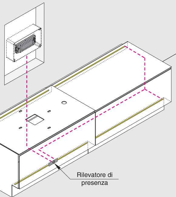
B Accensione / spegnimento luci di cortesia con rilevatore di presenza
