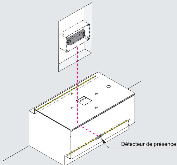
B Allumer/éteindre les lumières de courtoisie avec détecteur de présence
