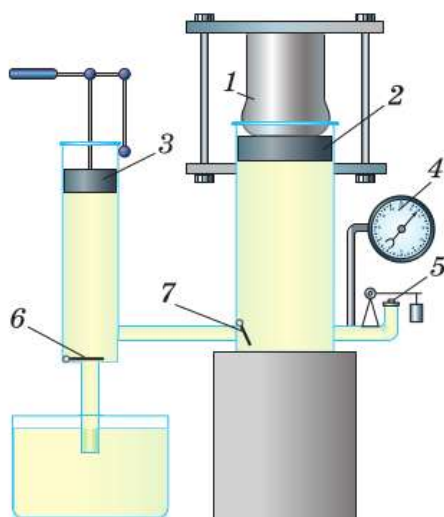
Рис. 148. Устройство гидравлического пресса
