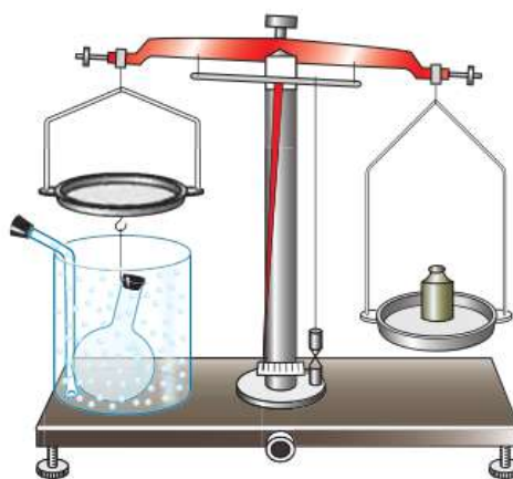
Рис. 153. Обнаружение силы, выталкивающей тело из газа
