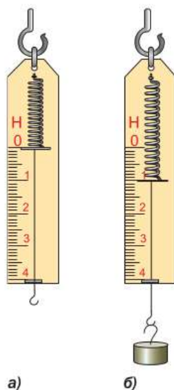
Рис. 77. Принцип действия динамометра
