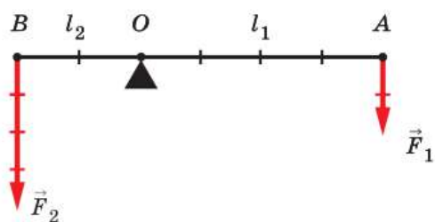
Рис. 171. Графическое изображение рычага с осью вращения
