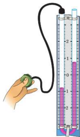
Рис. 141. Изменение уровня жидкости в коленах манометра
