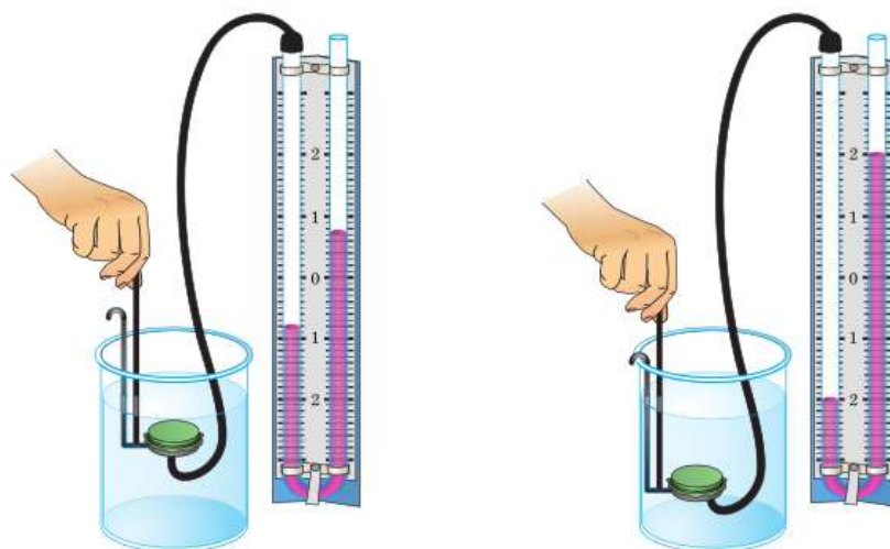
Рис. 142. Измерение давления жидкостным манометром
