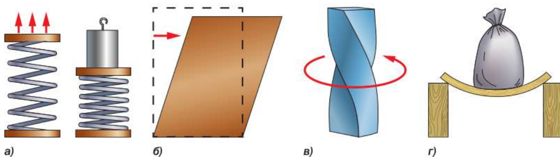
Рис. 68. Виды деформации:
