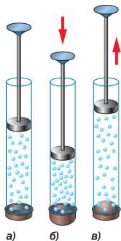
Рис. 101. Изменение давления газа при изменении его объёма
