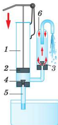
Рис. 146. Поршневой жидкостный насос с воздушной камерой
