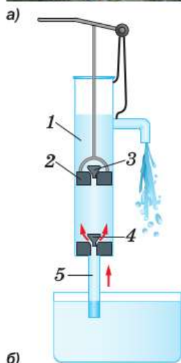
Рис. 145. Колонка с поршневым жидкостным насосом: а — внешний вид; б — устройство
