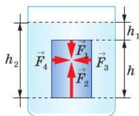
Рис. 151. Силы, действующие на погружённое в жидкость тело
