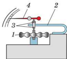
Рис. 138. Устройство барометра-анероида
