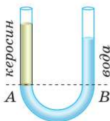
Рис. 123. Жидкости разной плотности устанавливаются на разных уровнях
