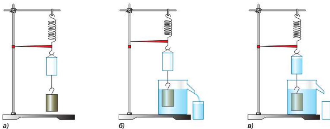
Рис. 154. Опыты с ведром Архимеда
