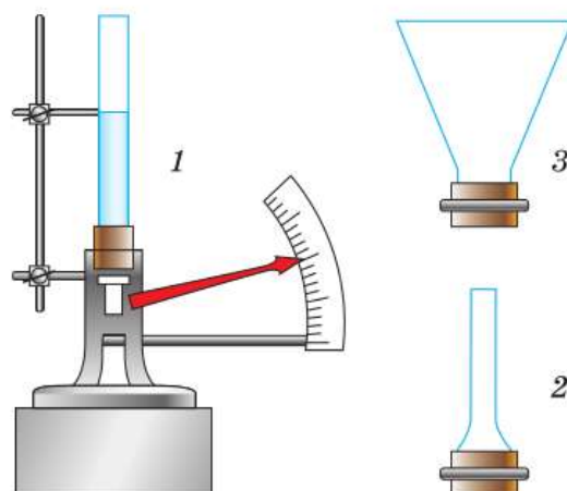
Рис. 118. Экспериментальная проверка гидростатического парадокса
