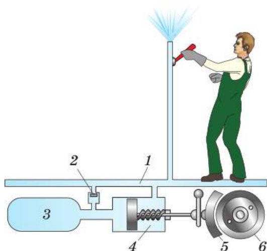
Рис. 109. Устройство пневматического тормоза
