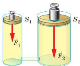
Рис. 147. Принцип действия гидравлической машины
