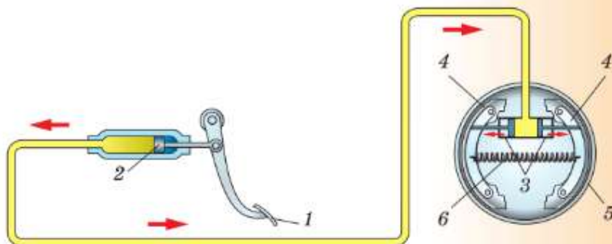
Рис. 150. Схема автомобильного гидравлического тормоза
