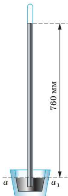
Рис. 133. Опыт Торричелли
