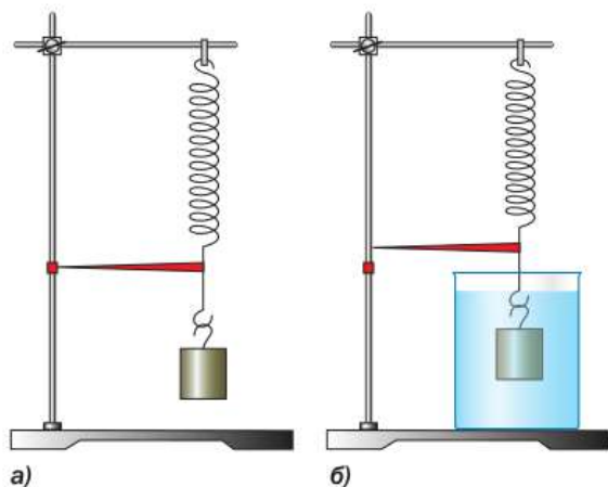
Рис. 152. Обнаружение силы, выталкивающей тело из жидкости
