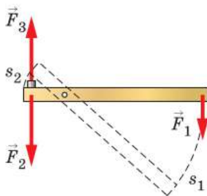
Рис. 186. Выигрываем в силе, но проигрываем в расстоянии
