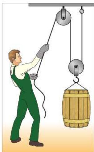
Рис. 185. Комбинация подвижного и неподвижного блоков — полиспаст
