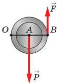
Рис. 184. Подвижный блок как рычаг с неравными плечами
