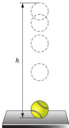
Рис. 191. При падении потенциальная энергия мяча превращается в кинетическую
