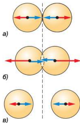
Рис. 69. Силы взаимодействия молекул при их сближении и удалении: красными стрелками показаны силы отталкивания, синими — притяжения
