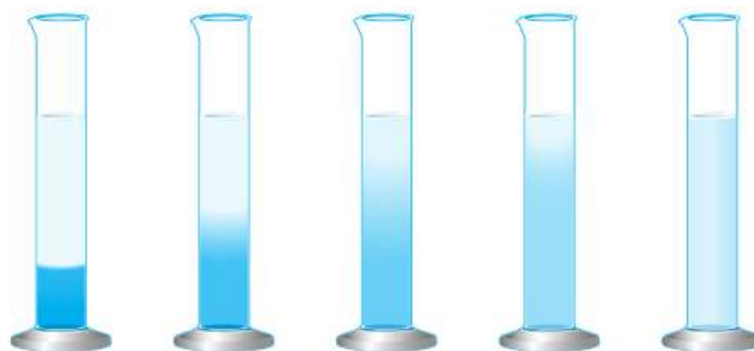
Рис. 26. Диффузия в жидкостях: взаимное проникновение воды и раствора медного купороса друг в друга
