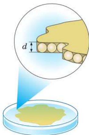
Рис. 25. Масляная плёнка на поверхности воды
