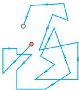
Рис. 37. Траектория движения молекулы
