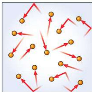
Рис. 99. Хаотическое движение молекул газа
