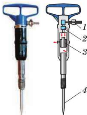
Рис. 108. Внешний вид и устройство пневматического отбойного молотка
