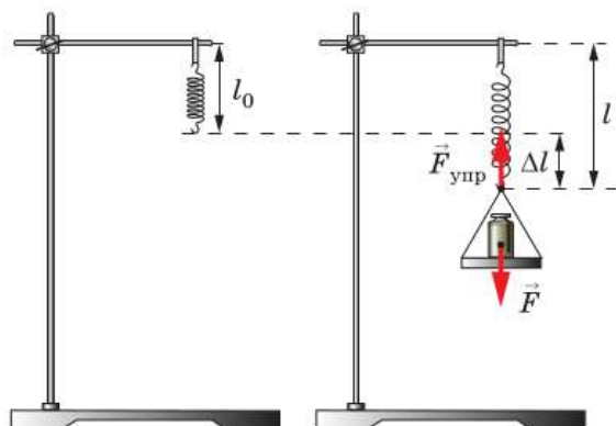
Рис. 71. Возникновение силы упругости при деформации
