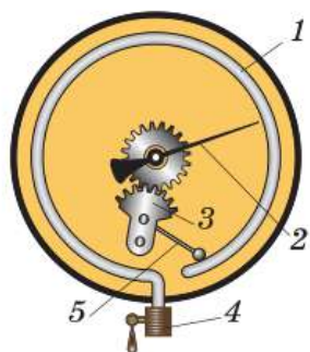
Рис. 144. Устройство металлического манометра
