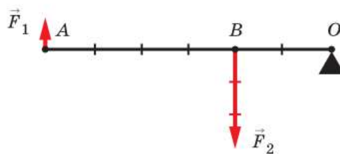
Рис. 172. Равновесие рычага второго рода
