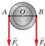
Рис. 182. Неподвижный блок как равноплечий рычаг
