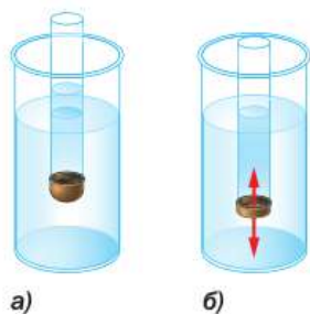
Рис. 111. Выпрямление плёнки при одинаковом уровне воды в трубке и в сосуде
