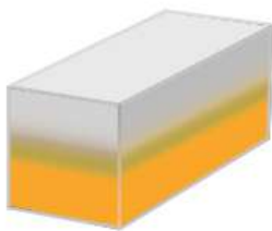
Рис. 28. Диффузия в твёрдых телах
