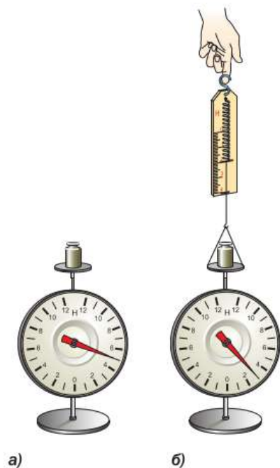
Рис. 84. Нахождение равнодействующей двух сил, действующих на тело в противоположные стороны
